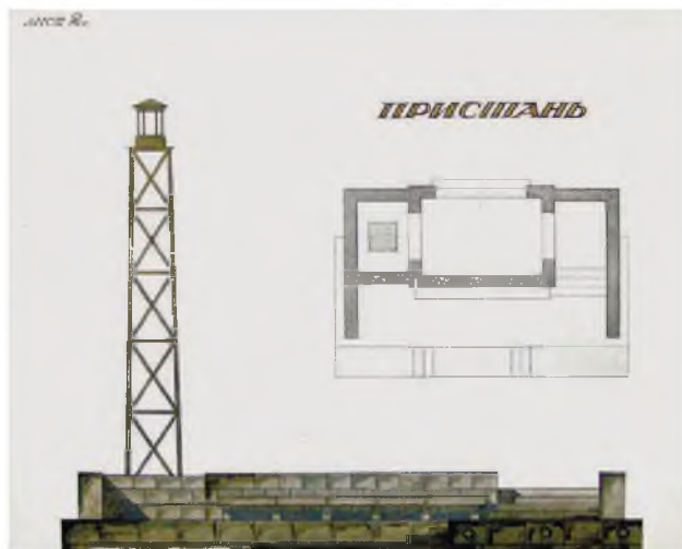
Проект пристани. Арх. Н. Б. Борисов 1925 г. Историко-культурный музейный комплекс в Разливе
