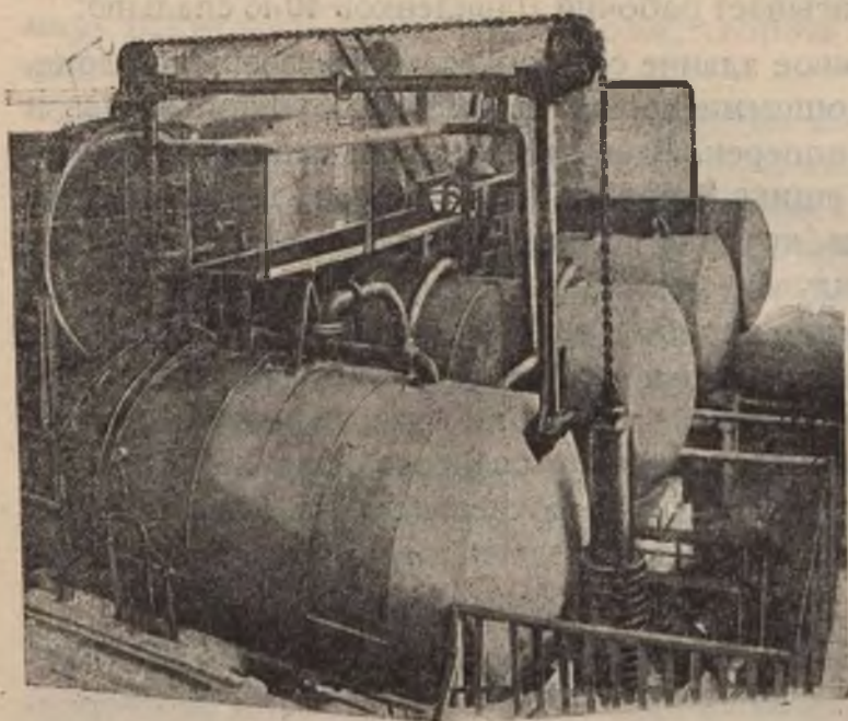
После проведения в жизнь предложения слесаря т. Шестопалова крышка куба „Матер-платт“ поднимается механически мотором. Раньше ее подымали вручную 3—4 человека.
